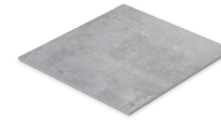
Boden- und Wandfliese 60 x 60 cm Nexos grau matt (600 x 600 x 10 mm) rektifiziert Trittsicherheit R 10/B NX66.F02M
