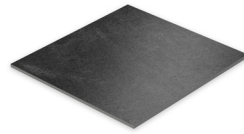
Boden- und Wandfliese 60 x 60 cm Nexos Stone anthrazit matt (598 x 598 x 9,5 mm) rektifiziert Trittsicherheit R 10/B NT66.F05M
